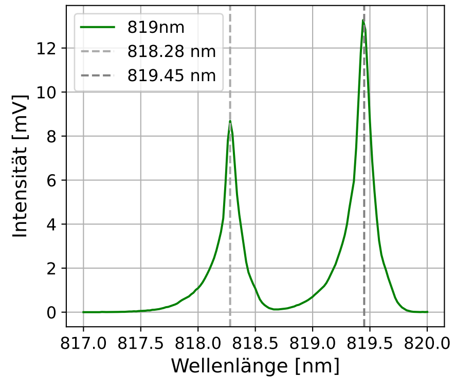
819 nm
