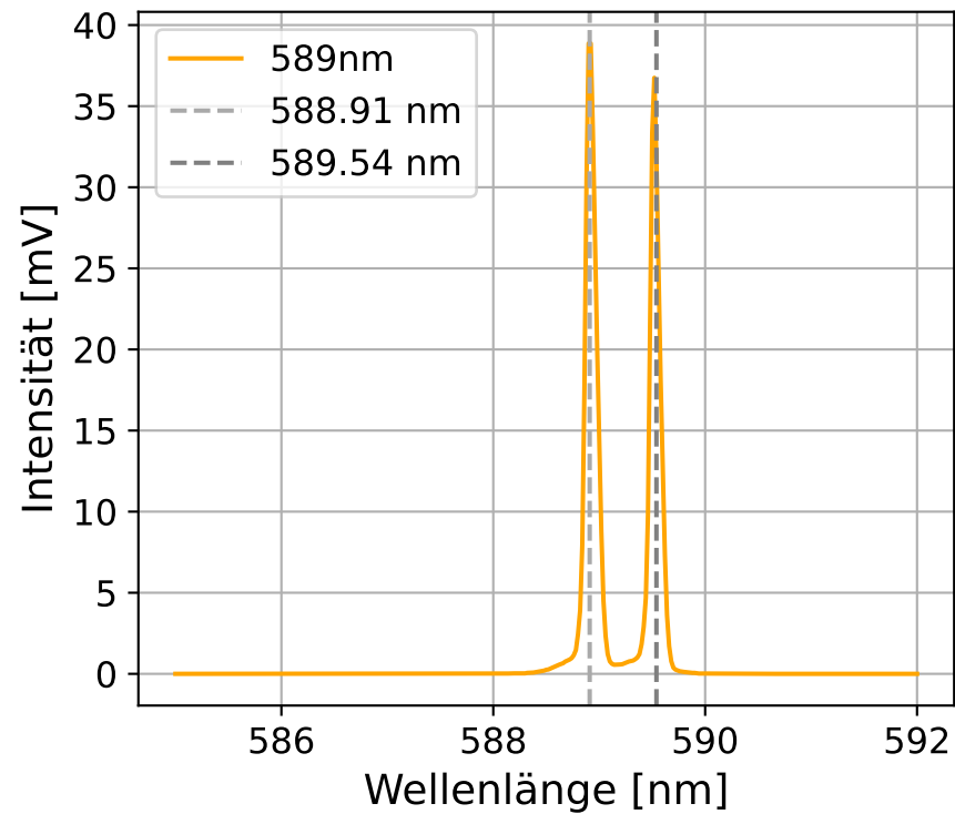
589 nm
