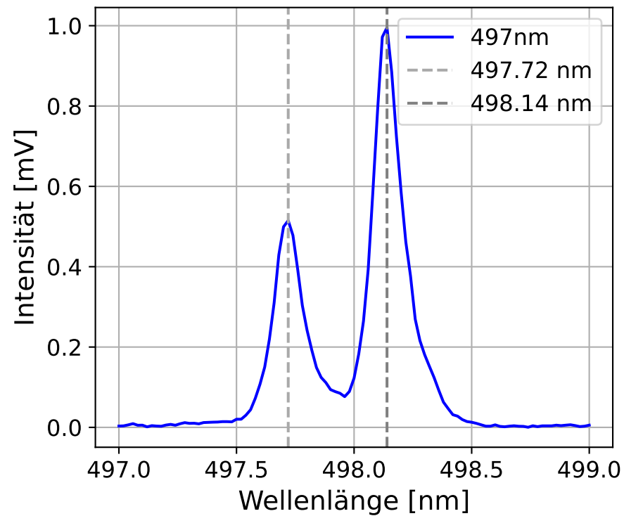
497 nm
